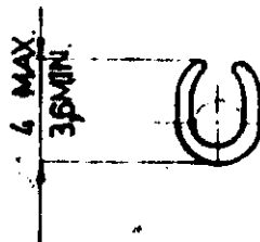
SECCION-AA
