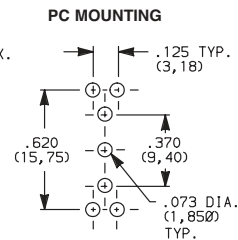
E112SD1_BE SPDT
