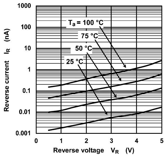
Fig. 8.2 I_R - V_R
