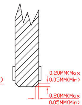
VIEW C-C OPTIONAL
