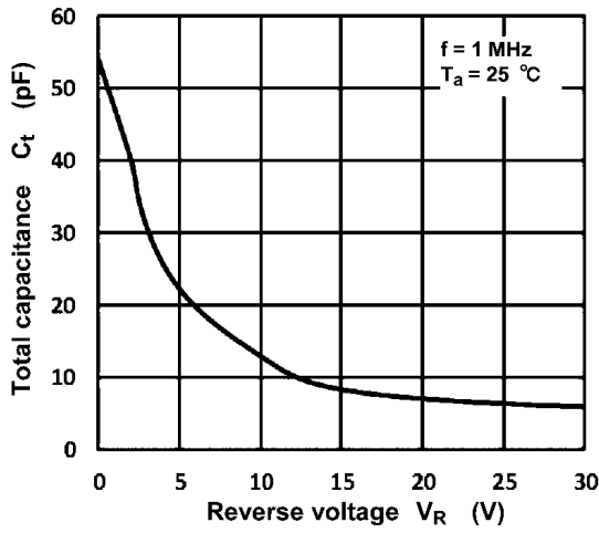
Fig. 8.3 C_t - V_R
