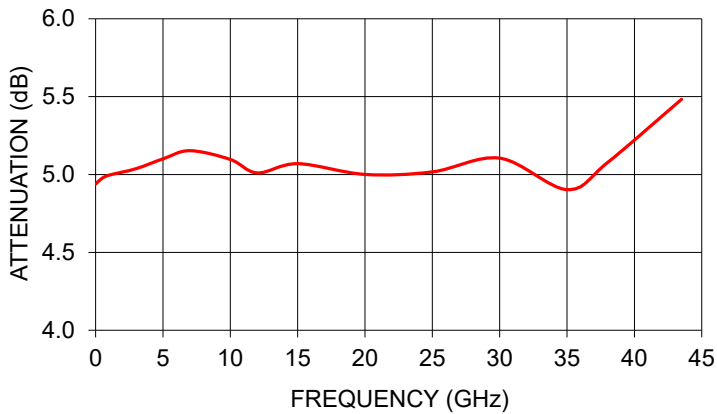
KAT-5+ ATTENUATION
