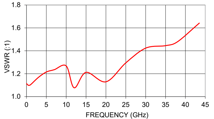
KAT-5+ VSWR
