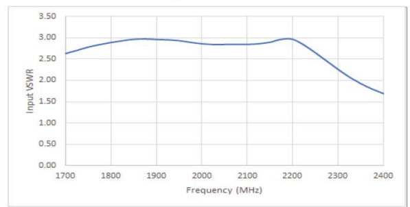
Input VSWR
