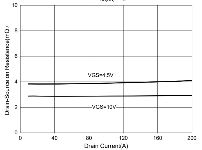
Fig. 4 - R_{DS(ON)} - I_D
