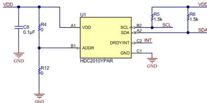
Figure 2. HDC2010EVM : Sensor Module
