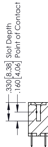
SECTION A-A
