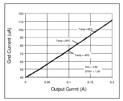
Fig. 45 IOOUT - IGND
