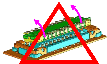
短手方向の斜め抜去
