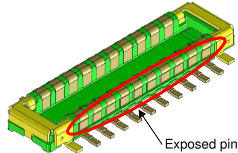
プラグ Plug PN: 505070-**20
