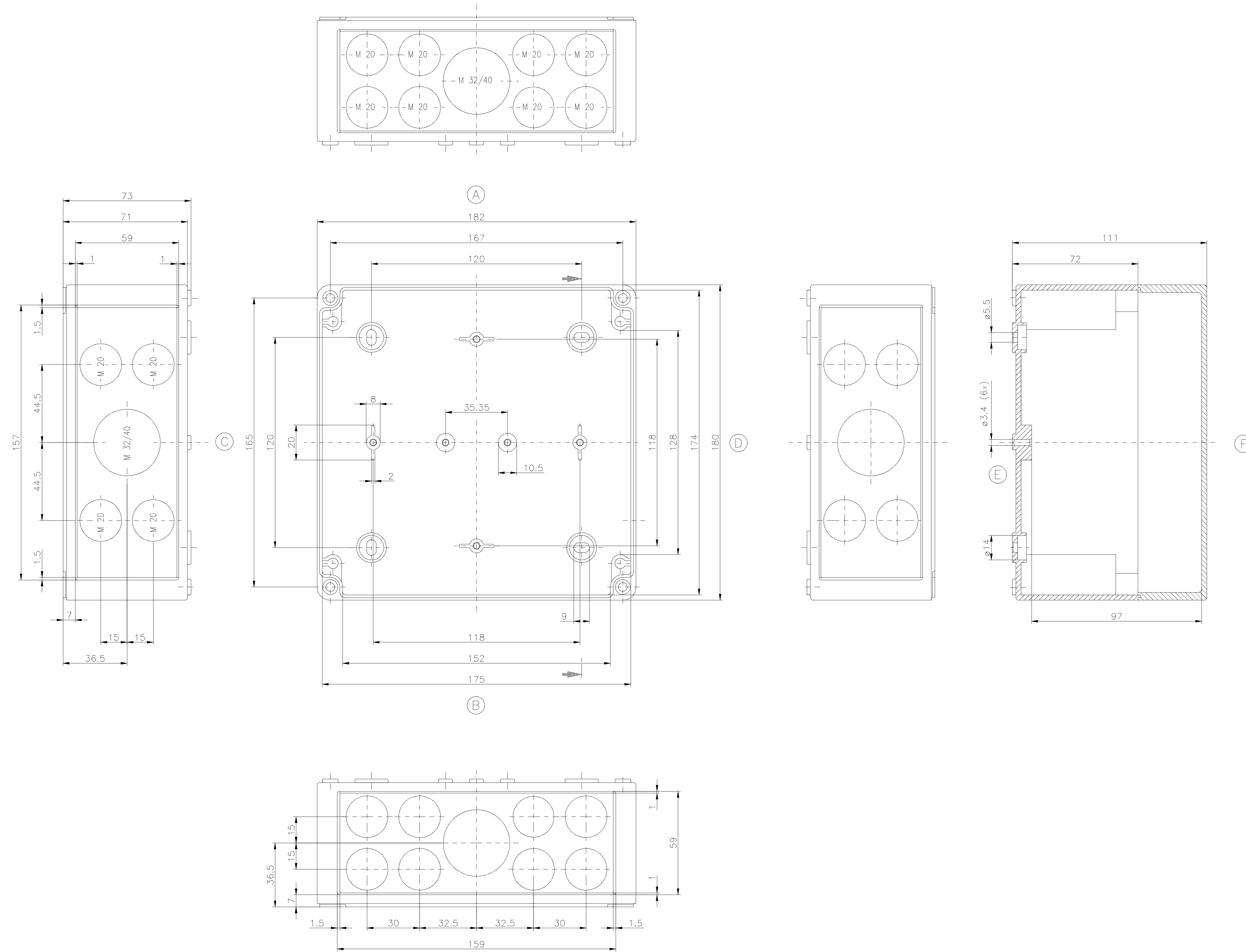
Kompaktgehäuse PCI 09-11M Bestell-Nr. 60.181825
