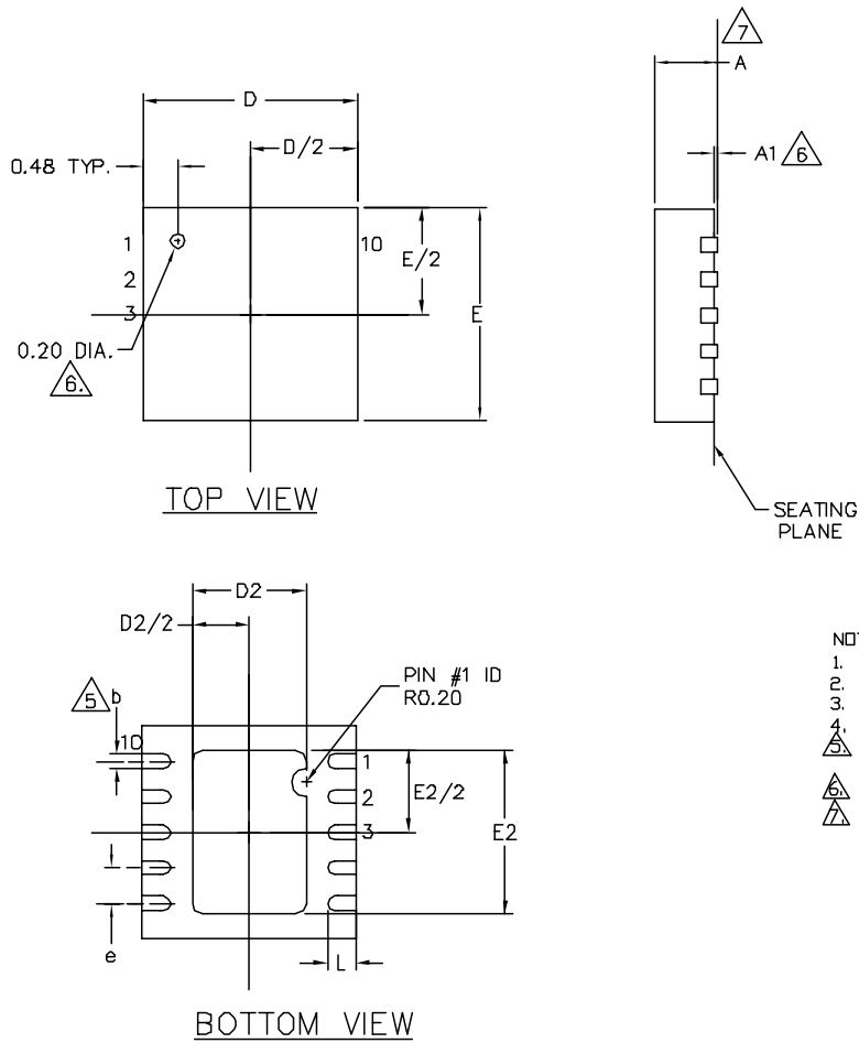
10-Pin 3x3 MLF (MLF)
