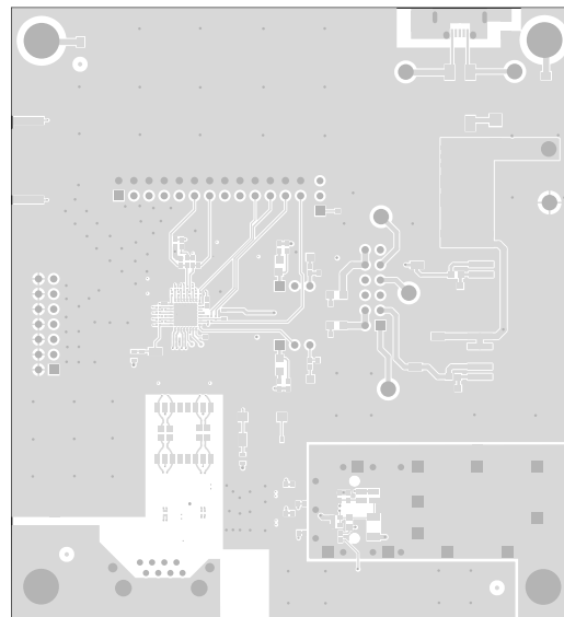
Figure 21. Top Layer
