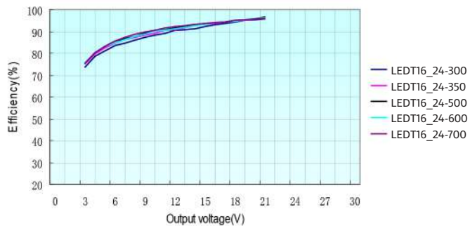
Vin=24V
