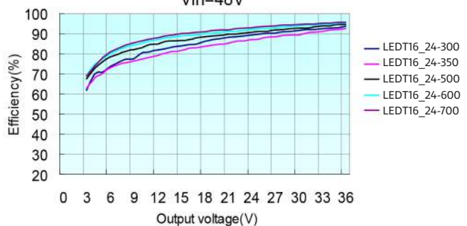
Vin=48V
