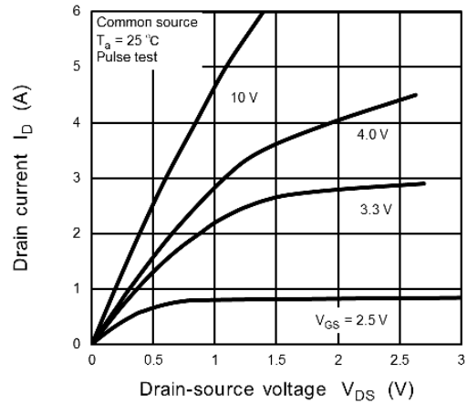
Fig. 7.2 I_D - V_{DS}
