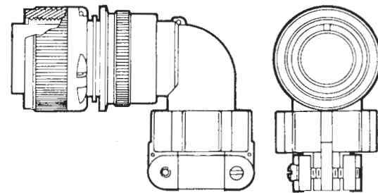
90° Angle plug MS 3108E and R/CA 3108E/F/R 1) 1) MS 3108R, CA 3108F/R without cable clamp
