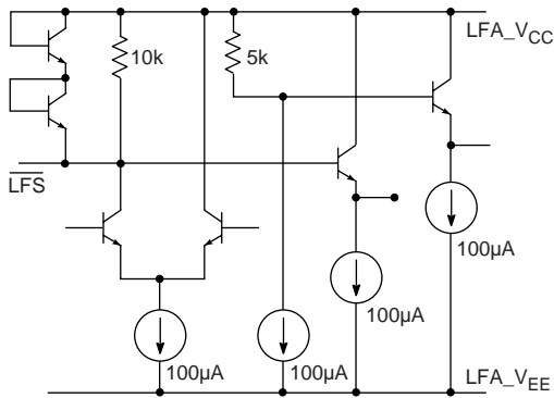
Fig. 7 \overline{\text{LFS}} Input
