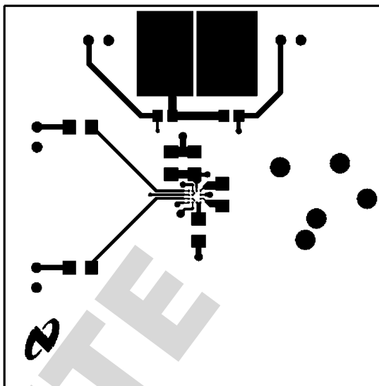
Top Layer
