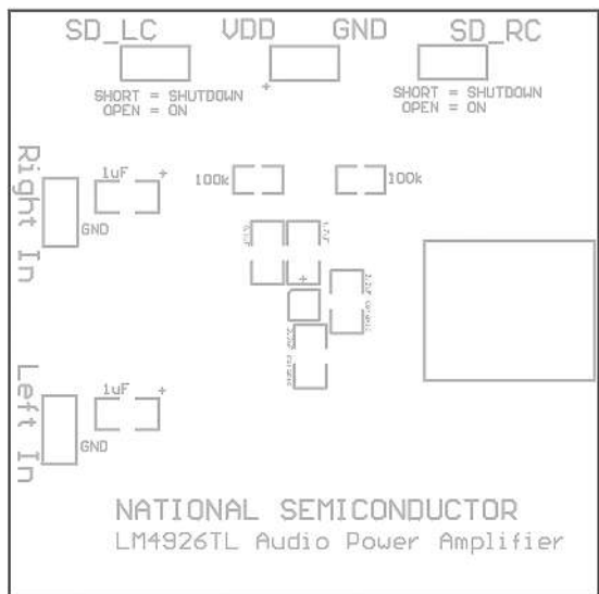
Top Overlay
