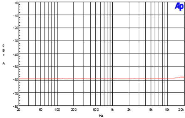
17. CMRR
