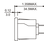
FAST-ON LUG
