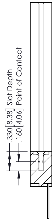
SECTION A-A
