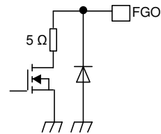
12) FGO pin
