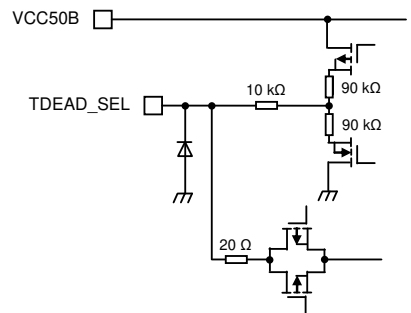
9) TDEAD_SEL pin
