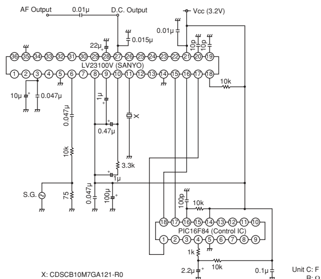
CDSCB10M7GA121-R0
