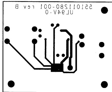
Bottom Layer
