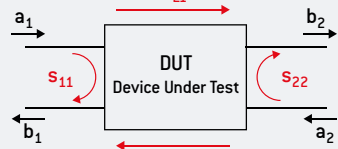
Figure 2: S parameters
