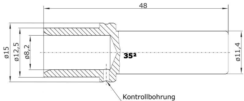
Hauptabmessungen Kontaktbuchse
