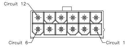
12PIN
