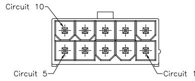
10PIN
