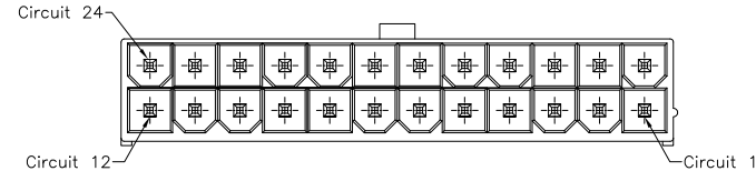
24PIN
