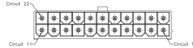
22PIN
