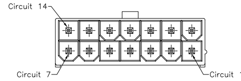
14PIN
