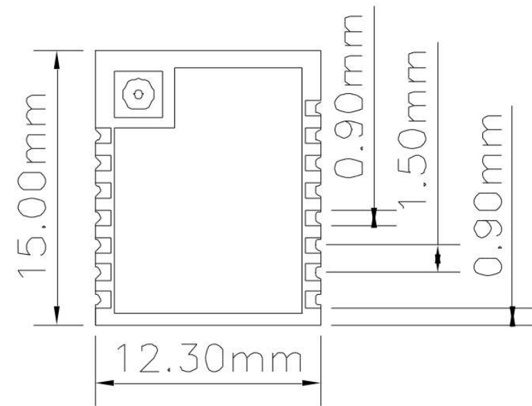
(a) 俯视图
