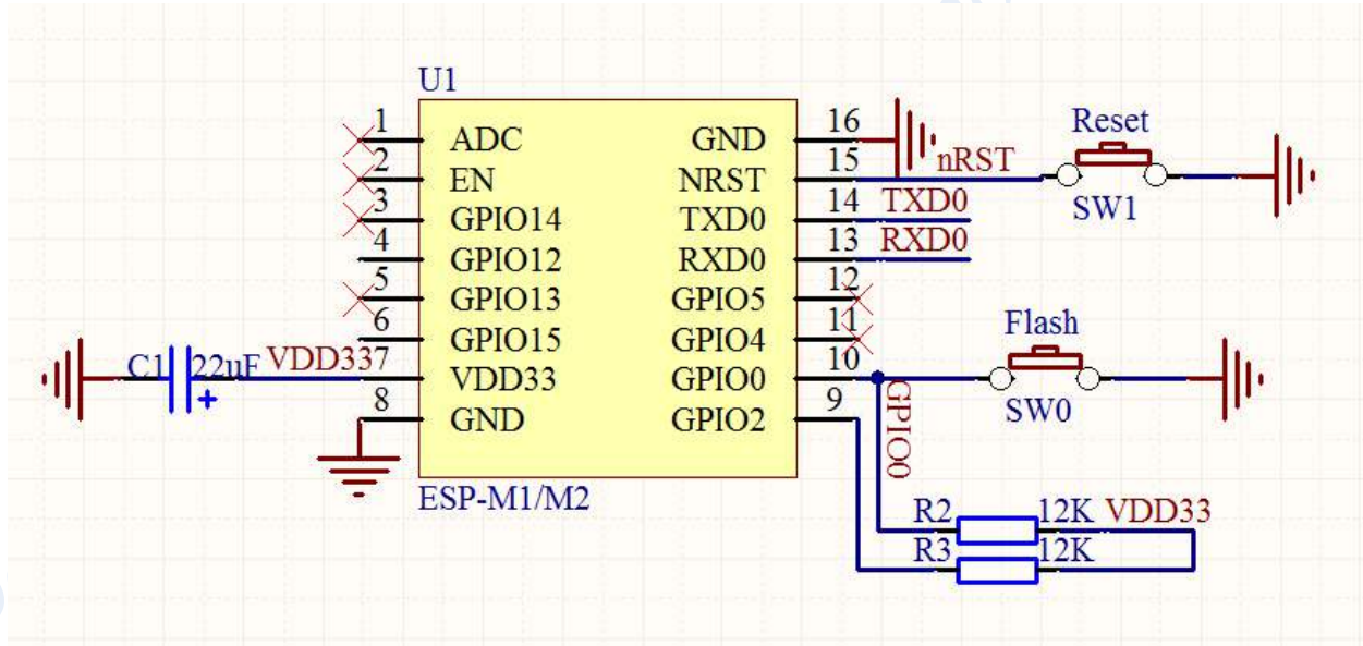
图 8.1 最小系统
