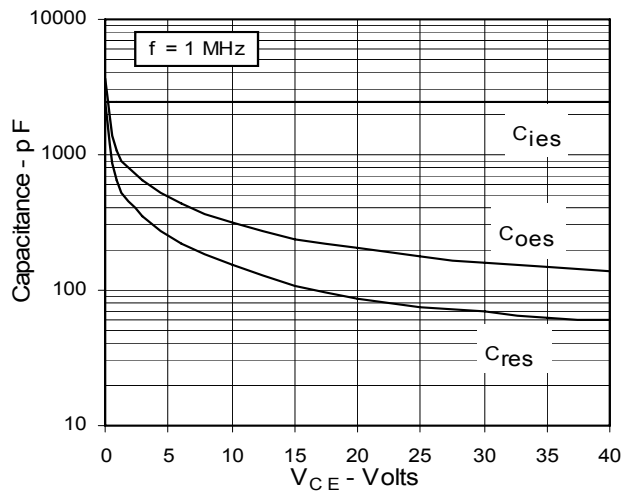
Fig. 15. Capacitance
