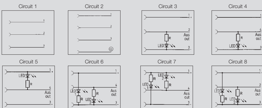
Wiring scheme
