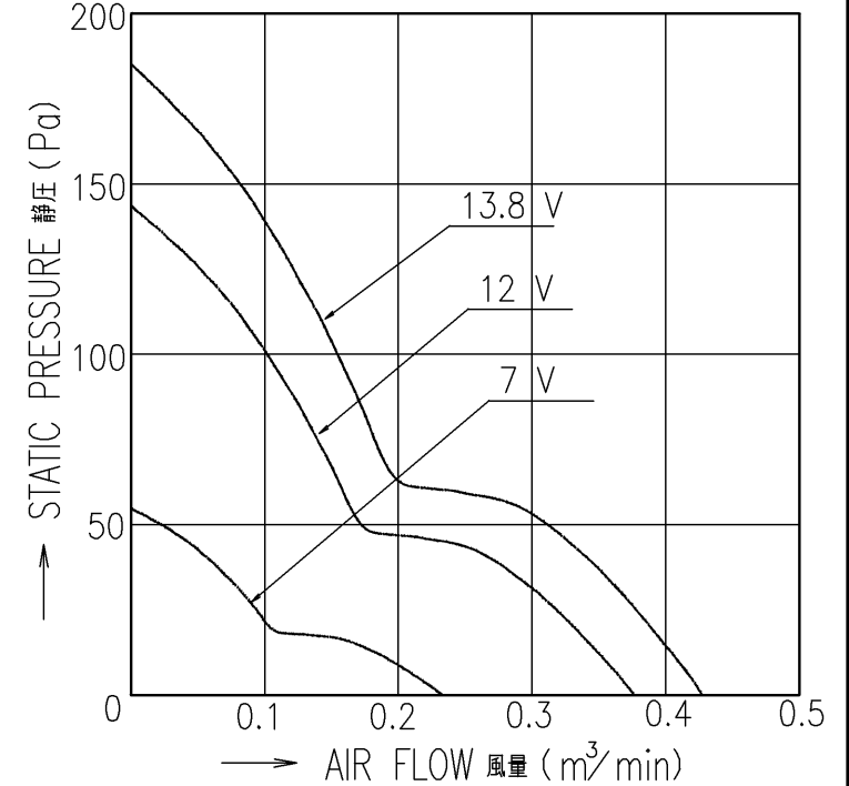
風量-静圧特性例
