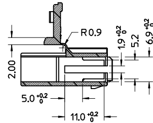
SEZ. B-B
