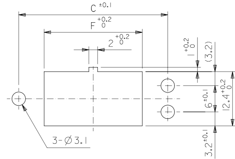
パネル切抜寸法 (参考)
