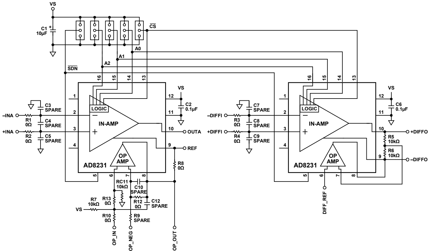
Figure 3. AD8231-EVALZ Schematic
