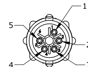
WIRING VIEW W18982-5SG-P-5XX
