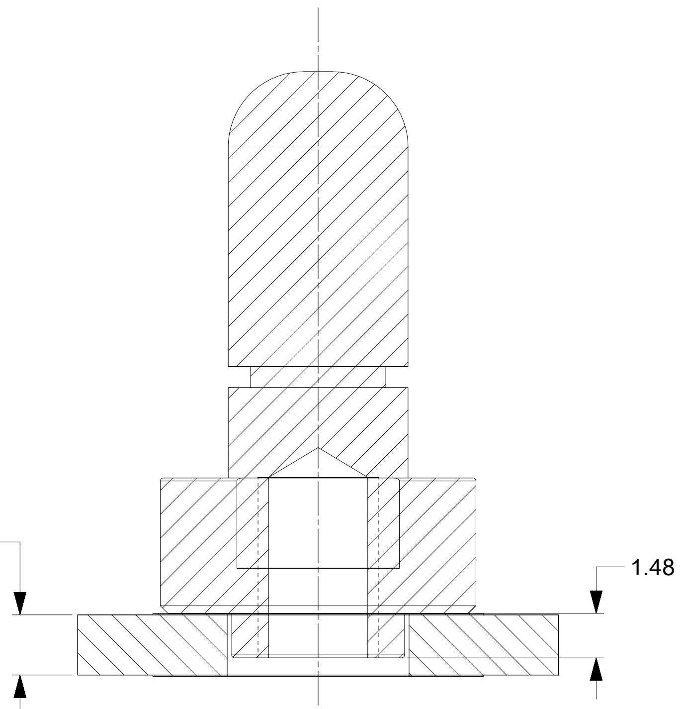
SECTION A-A
