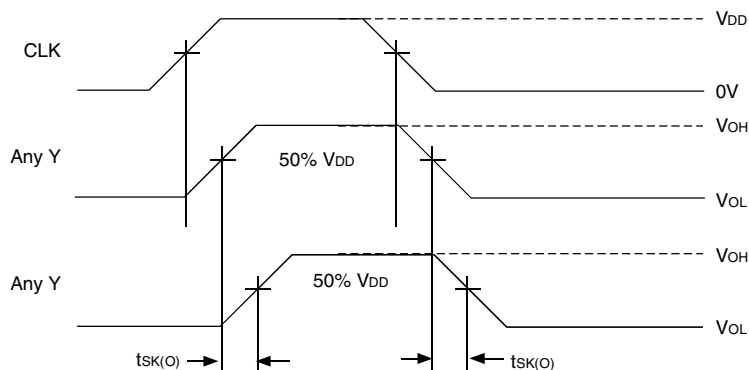
Output Skew
