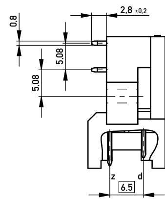
Bestückungsplan / contact layout
