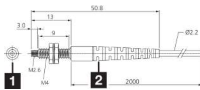
2) Kabelschutztülle
