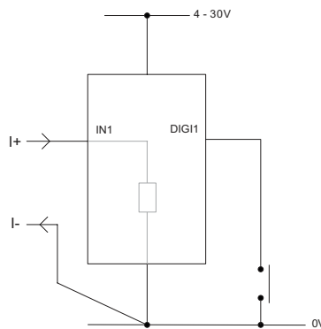
DIGITAL HOLD DIG1 will hold the display
