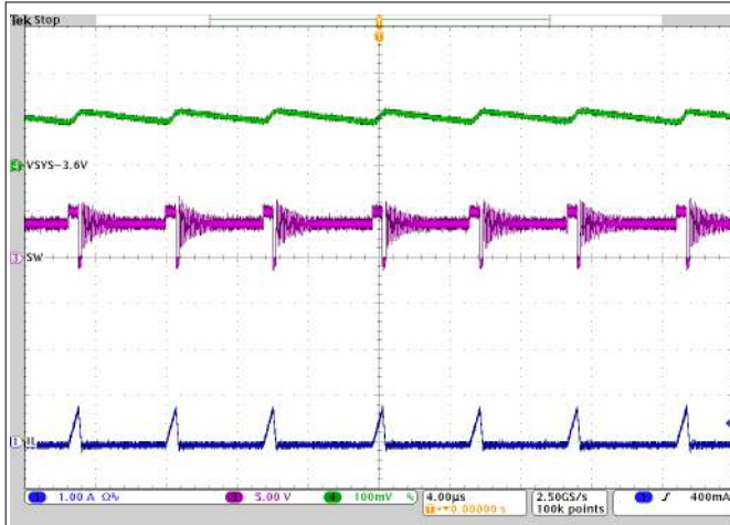
V_{BUS} = 5\text{ V} I_{SYS} = 50\text{ mA} Charge Disabled
