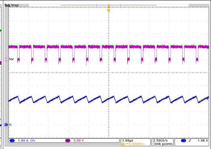
V_{BUS} = 5\text{ V} I_{CHG} = 2\text{ A} V_{BAT} = 3.8\text{ V}
