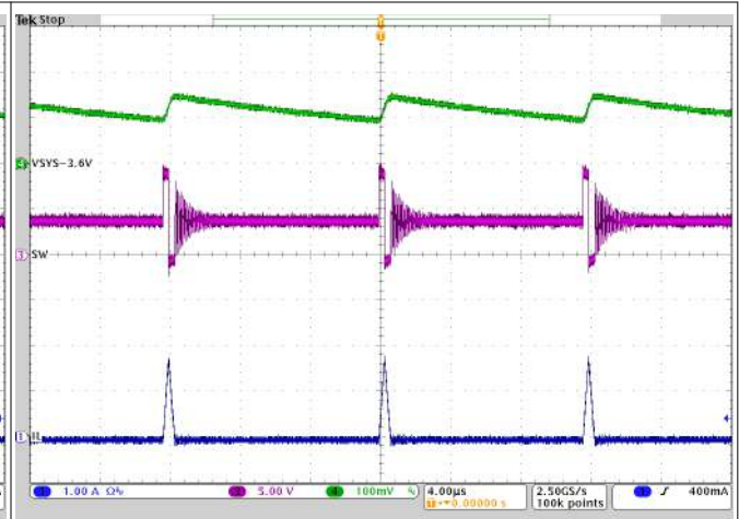
V_{BUS} = 9\text{ V} I_{SYS} = 50\text{ mA} Charge Disabled
