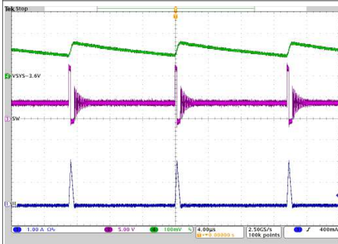
V_{BUS} = 12\text{ V} I_{SYS} = 50\text{ mA} Charge Disabled
