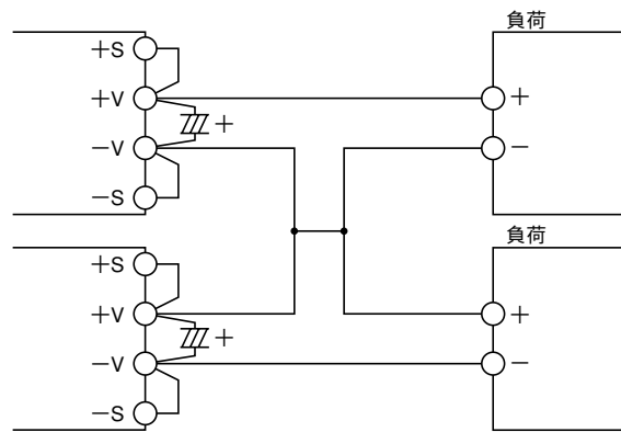
図12-2 正出力使用の直列運転
