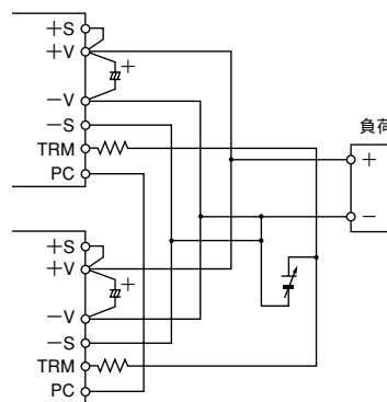
図3-4 外部電圧印加による出力電圧可変が可能な並列運転
