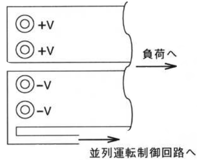
図3-4 -V配線例
