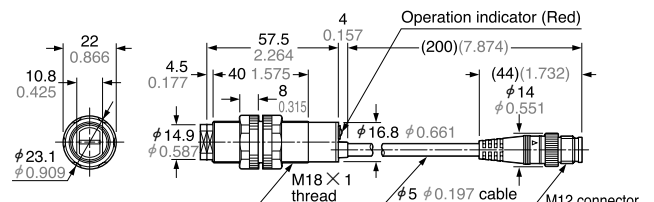
CY-29-J Sensor
