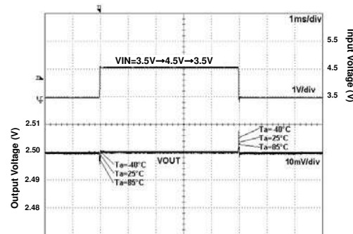
Fig 128. VIN Response
