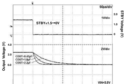
Fig 127. Discharge Time
