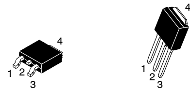
DPAK CASE 369C STYLE 2
