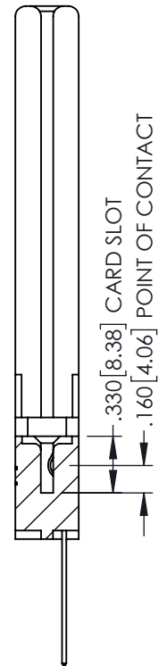
SECTION A-A
