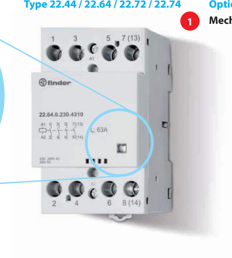
Type 22.44 / 22.64 / 22.72 / 22.74
