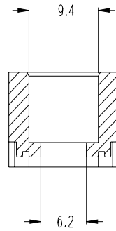
SEZIONE A-A
